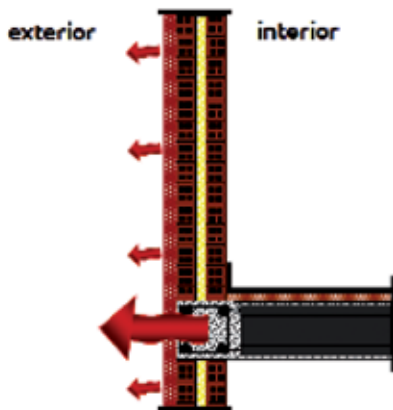
Figura 8: Afectación puentes térmicos en función a la tipología de vivienda.
