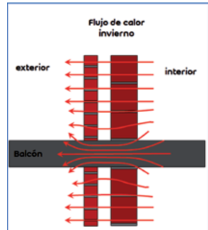
Figura 4: Flujo de calor en cerramiento con puente térmico.
